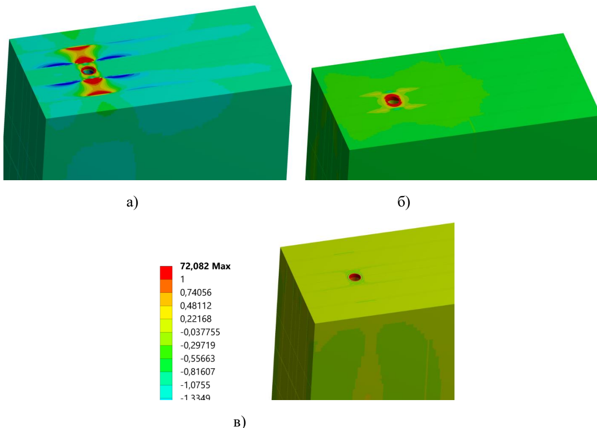
Рис. 3. Характер розподілу нормальних напружень для зразка з розташуванням вклеєного стержня за схемою 1: а – нормальні напруження по осі X; б – нормальні напруження по осі Y; в – нормальні напруження по осі Z
