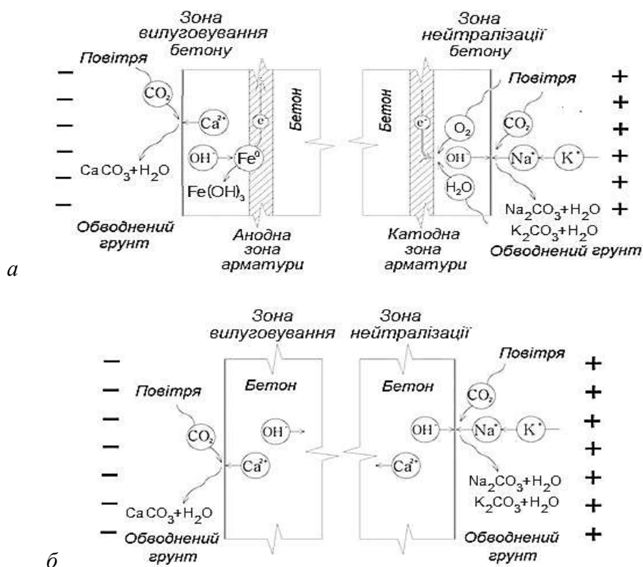
Рис. 8. Схема протікання струму через конструкції високих пасажирських платформ: а – залізобетонні стояки (рис. 1, а); б – бетонні опори (рис. 1, б)
