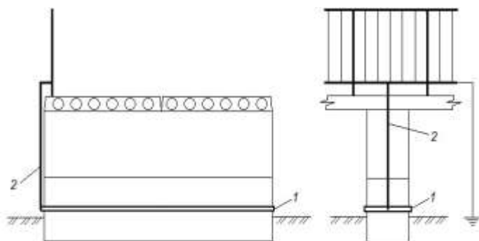
Рис. 12. Конструктивно-технологічне рішення захисту опори пасажирської платформи з заземленим екраном з електропровідної композиції:
