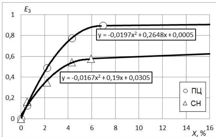
Рис. 10. Залежність показників ефективності захисту E_p із заземленими екранами з електропровідних композицій на основі портландцементу ПЦ і силікату натрію СН від площі контакту сталевго заземлювача з екраном X
