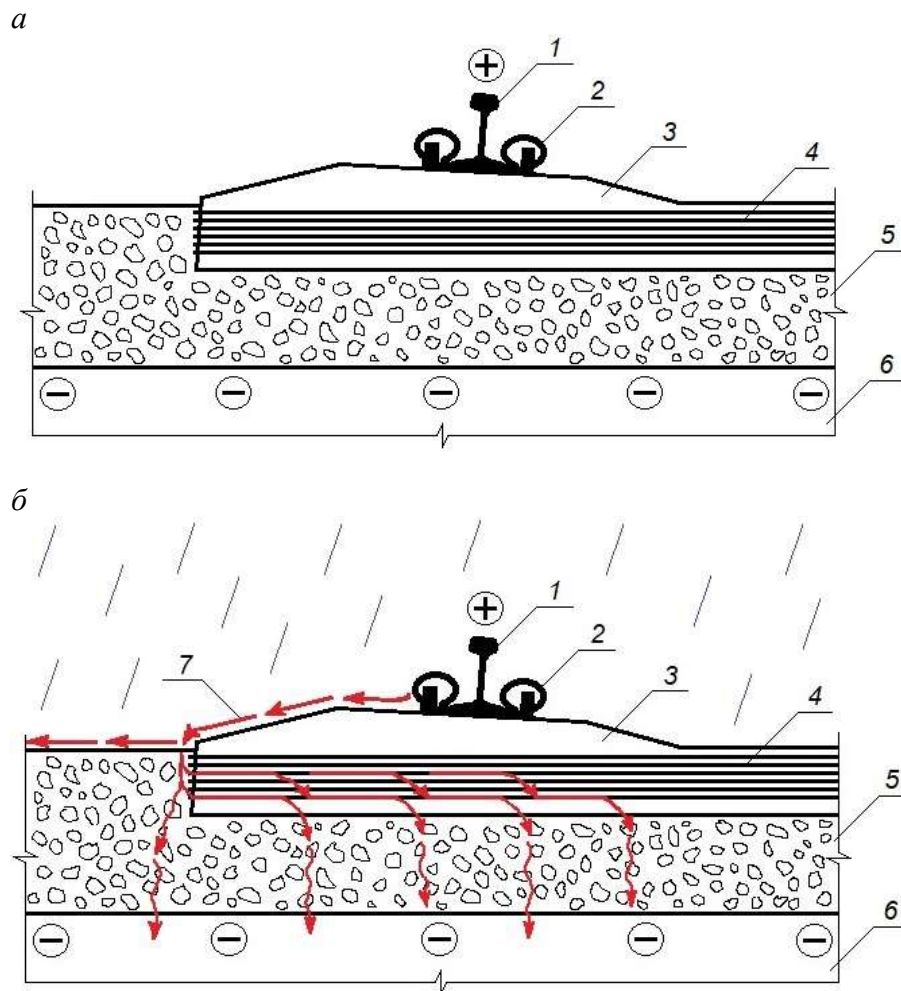
Рис. 6. Схема протікання струму витoku через шпали та баласт: а – у суху погоду (струмом можна знехтувати); б – під час атмосферних опадів: 1 – рейка; 2 – рейкове скріплення; 3 – бетон шпали; 4 – арматурний дріт; 5 – баласт; 6 – земляне полотно; 7 – струм витoku
