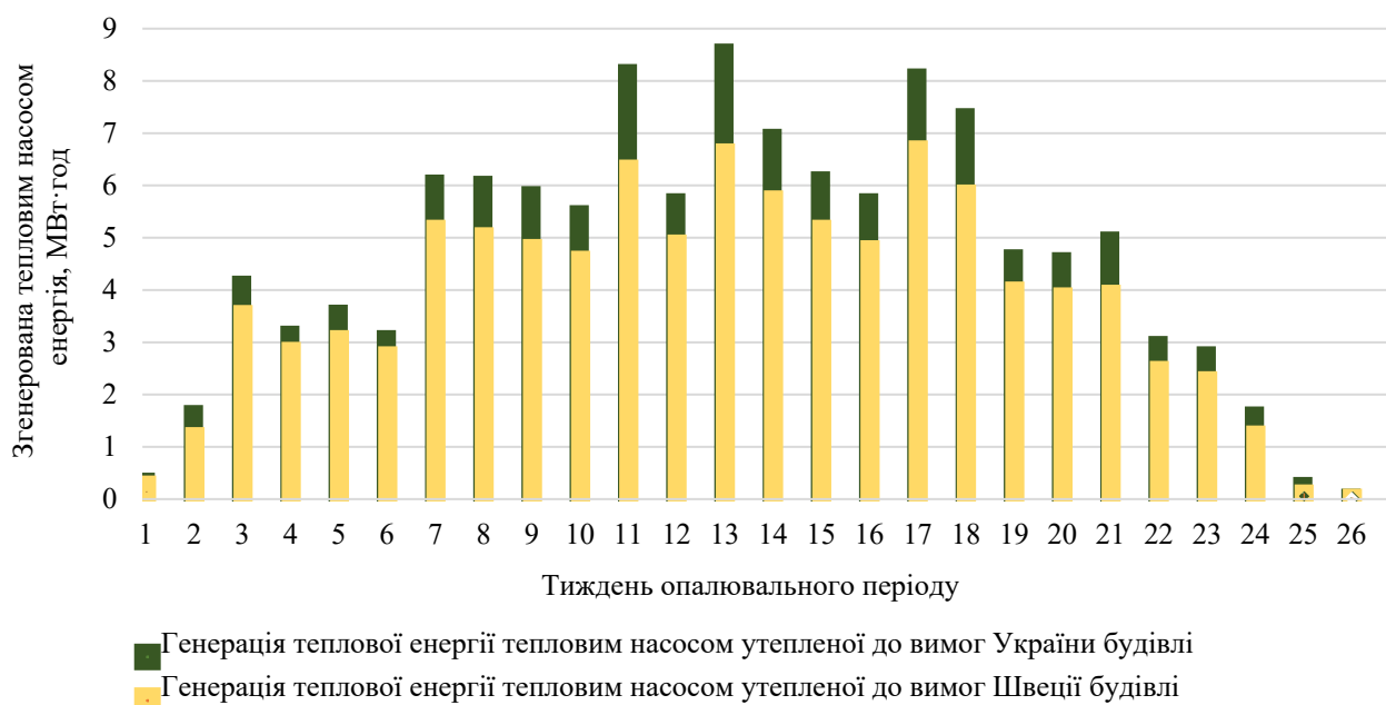
Рис. 5. Генерація теплової енергії тепловим насосом протягом опалювального періоду при покращенні теплової оболонки будівлі відповідно до вимог України і Швеції
