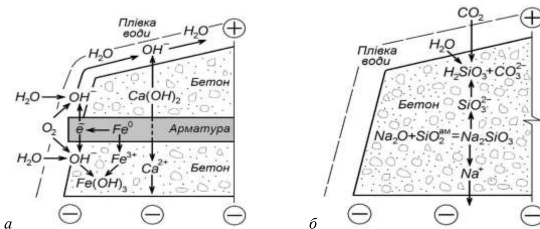
Рис. 7. Схема протікання струму через бетон і арматуру шпали та корозійних процесів: а – протікання струму через бетон і арматуру та електродокорозія арматури; б – інтенсифікація корозії бетону від ASR
