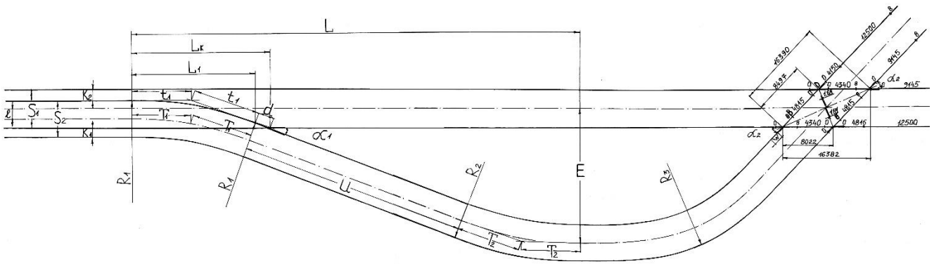
Рисунок 11.6 – Схема сплетіння колій 1520 і 1435 мм зі зміною сторонності
