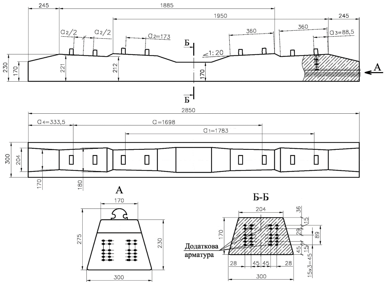
Рисунок В.4 – Залізобетонна шпала суміщеної колії 1520 мм і 1435 мм для рейок типу Р65 або UIC60 (60E1) і пружним скріплення
