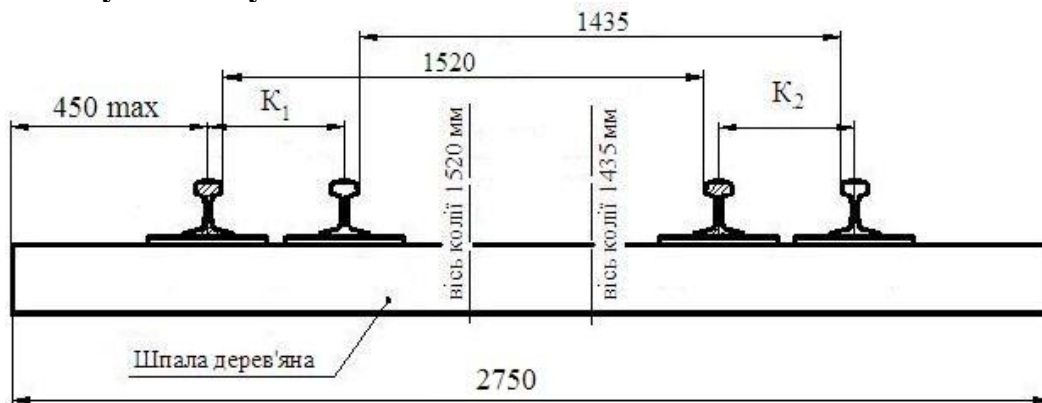
Рисунок 11.3 – Суміщена колія 1520 і 1435 мм на дерев'яних шпалах
