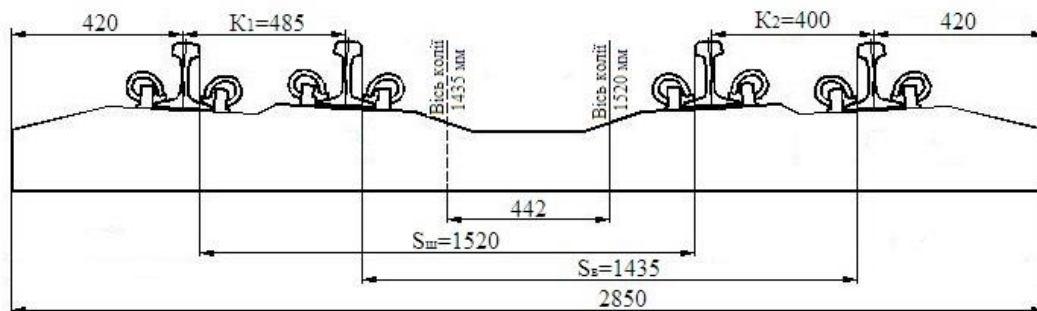
Рисунок 11.4 – Суміщена колія 1520 і 1435 мм на залізобетонних шпалах
