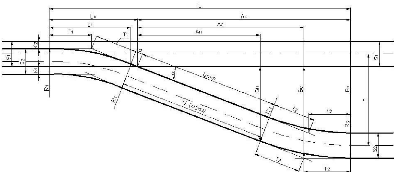
Рисунок 11.5 – Схема сплетіння колій 1520 і 1435 мм без зміни сторонності
