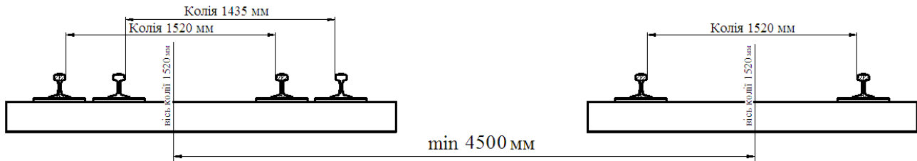
Рисунок 11.1 – Відстань між осями суміжних колій (суміщеної та колії 1520 мм)
