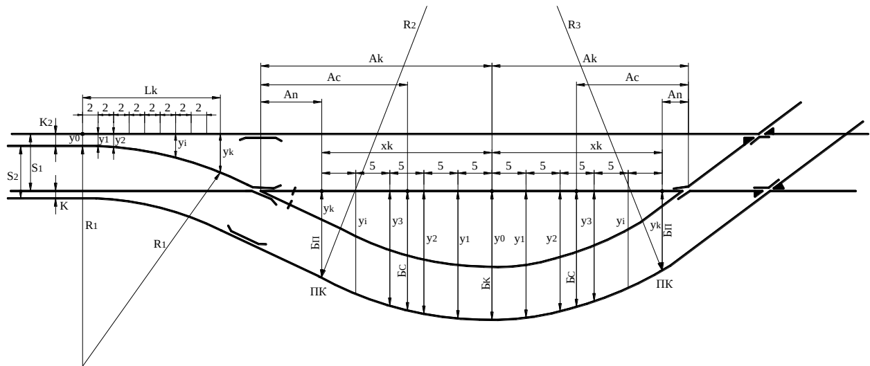
Рисунок 11.7 – Основні розміри захрестовинних кривих та схема розбивки ординат проміжних точок захрестовинних кривих
