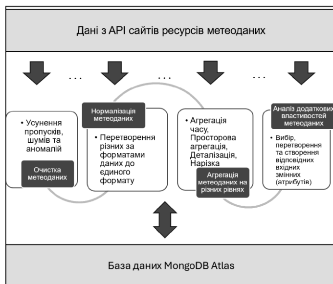
Рисунок 1. Підготовка метеоданих для навчання ML моделей
