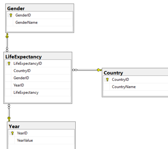
Рисунок 6. – Діаграма бази даних створенню за допомогою «ChatGPT 3.5»
