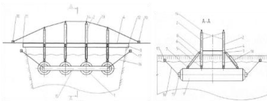
Рис. 1. Загальна схема понтонно-канатного мосту (викопіювання з патенту)
