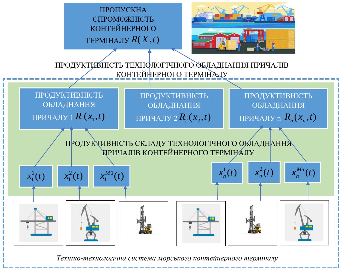
Рис. 2. Пропускна спроможність контейнерного терміналу як інтегральна характеристика відповідної техніко-технологічної системи
