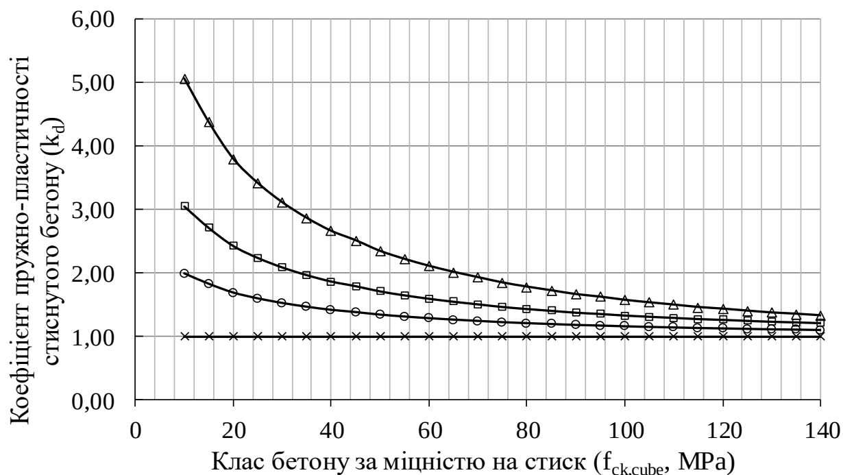
Рис. 3. Залежність коефіцієнта пружно-пластичності стиснутого бетону від його класу за швидкості деформування бетону:
