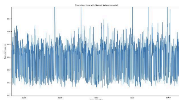
Рис. 2.18. Діагностична модель на основі нейронної мережі, реалізована в процесорі без графічного процесора: час обчислення для ковзних вікон
