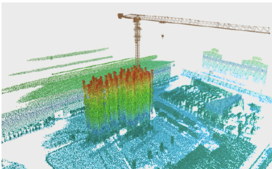
Рис. 1.8. 3д модель робочого простору крана та навколишніх об'єктів
