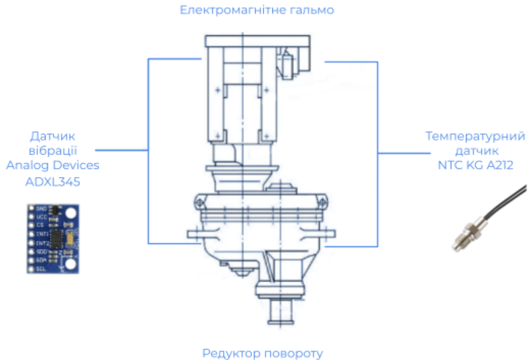
Рис. 2.7. – Схема розташування датчиків
