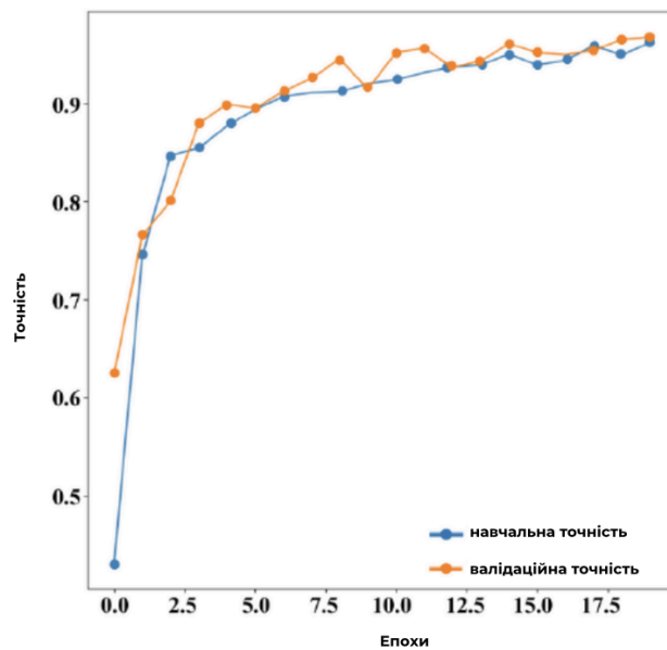
Рис. 4.4. Графік залежності функції точності від кількості епох
