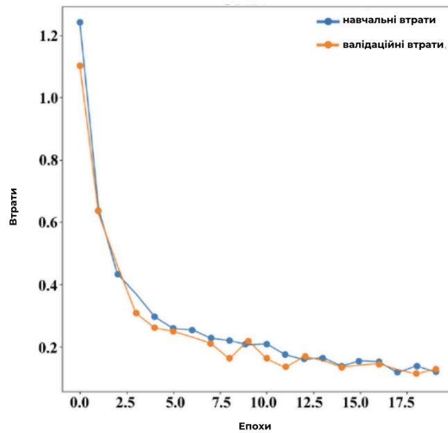
Рис. 4.3. Графік залежності функції втрат від кількості епох
