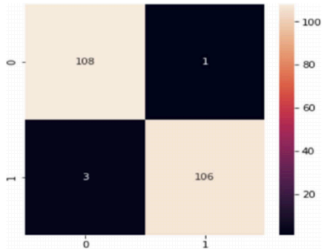
Рис. 4.5. Матриця невідповідностей моделі згорткової нейронної мережі
