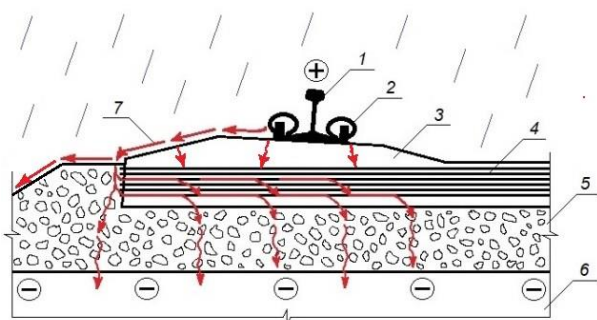
Рис. 2. Схема протікання струму витоку у дощову погоду крізь шпалу: 1 – рейка; 2 – рейкове скріплення; 3 – бетон шпал; 4 – арматурний дрiт; 5 – баласт; 6 – земляне полотно; 7 – струм витоку
